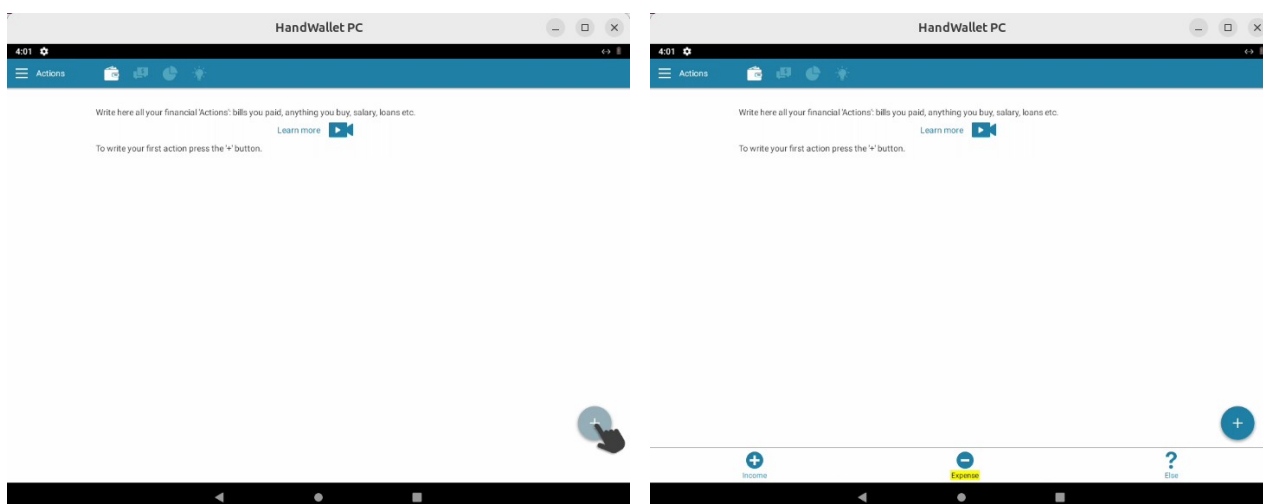
Сурет 11: Алғашқы әрекетке дейінгі «Actions» экраны (сол жақ). + басқаннан кейін әрекет түрін таңдаңыз (оң жақ).
