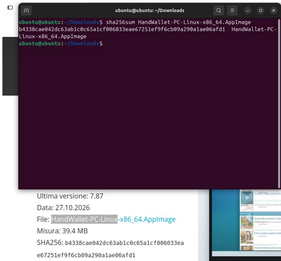
Figura 3: Nel Terminale: la firma calcolata. Sotto, nella pagina di download: la firma pubblicata. Sono identiche.
