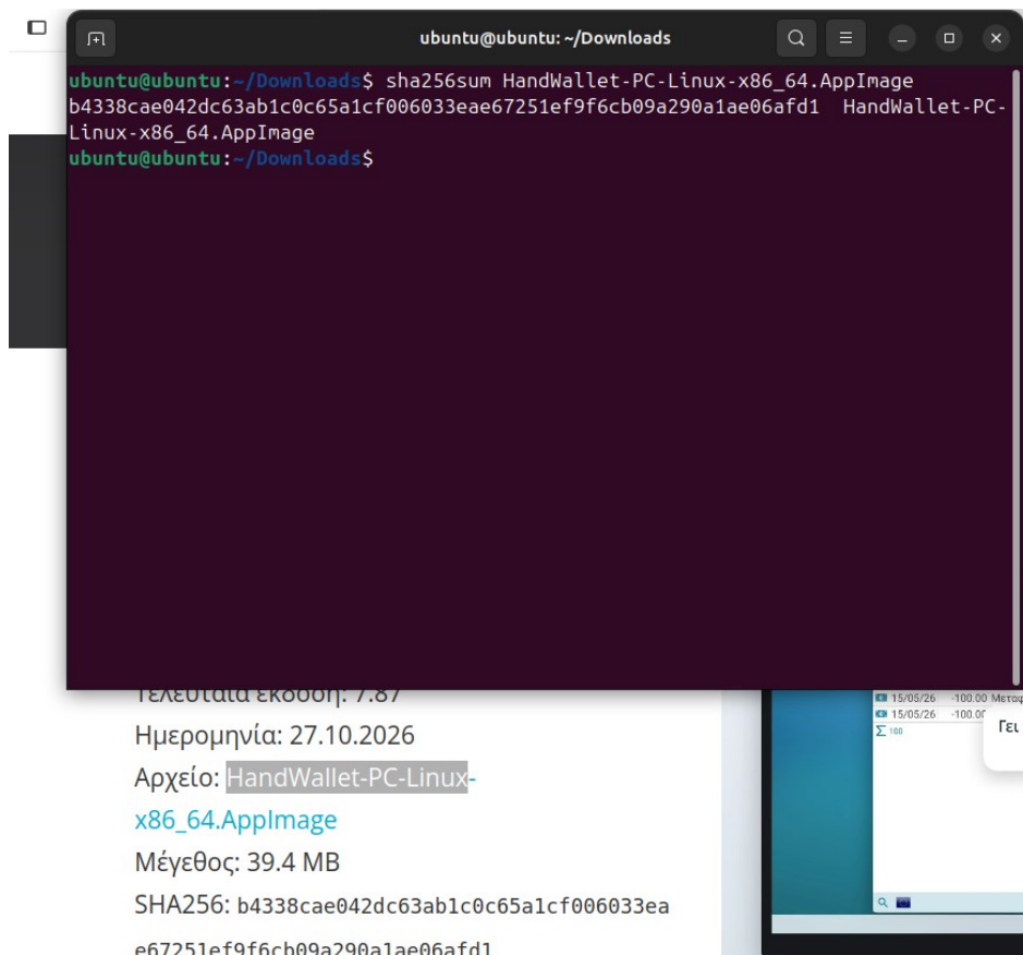
Εικόνα 3: Στο Τερματικό: η υπογραφή που υπολογίστηκε. Από κάτω, στη σελίδα λήψης: η υπογραφή που δημοσιεύσαμε. Είναι ίδιες.
